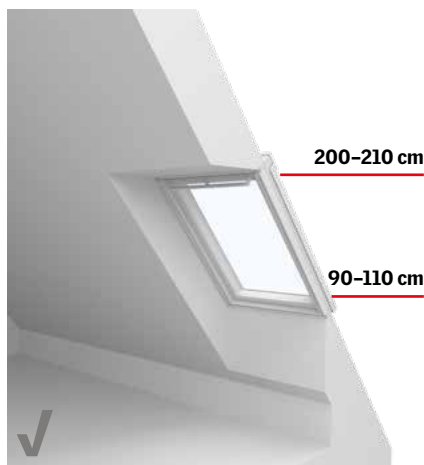
Optimálna výška nadmurovky
